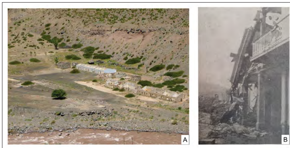
Figura 4. Daños ocasionados por el IDLOF del 10 de enero de 1934. (A). Fotografía tomada desde la ruta (RN 7) hacia el este donde se observan las ruinas de la estación de trenes, ubicada a 80 km del lago temporal. (B) Vista hacia el sur de los daños ocasionados en el hotel de Cacheuta, ubicado 150 km aguas abajo del lago temporal. Este sector del valle registró los mayores daños debido a la destrucción total de la central hidroeléctrica y del hotel y el registro de víctimas mortales.
